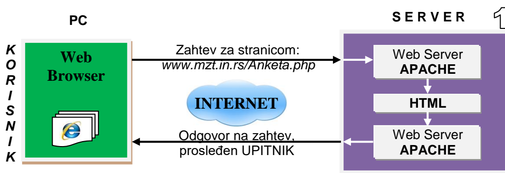
Slika 1 – Blok dijagram povezivanja zahteva korisnika sa odgovorom servera
