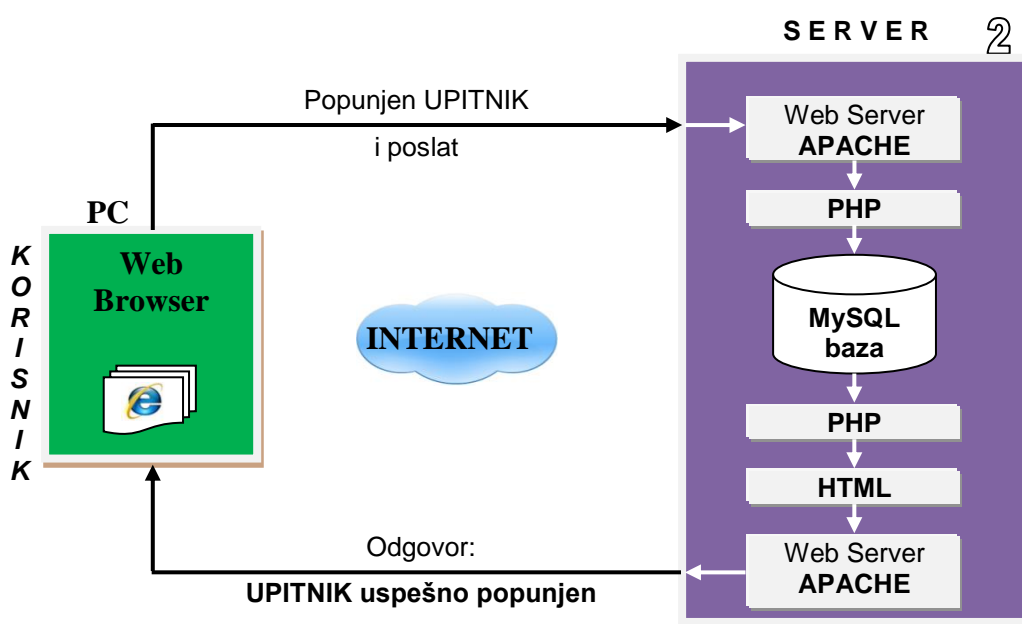
Slika 2 – Blok dijagram povezivanja poslatog upitnika sa bazom podataka
